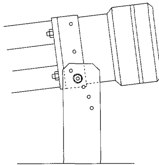
下向き5°の取付例
